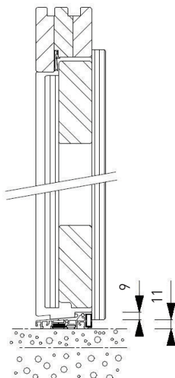
T20 Profilschwelle nach innen aufgehend
