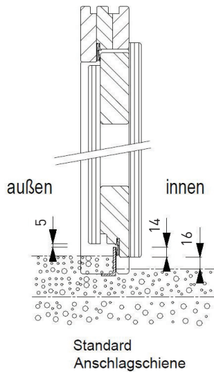
T20 beidseitig verschalt nach innen aufgehend
