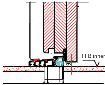
Profilschwelle für nach innen öffnende Türen
