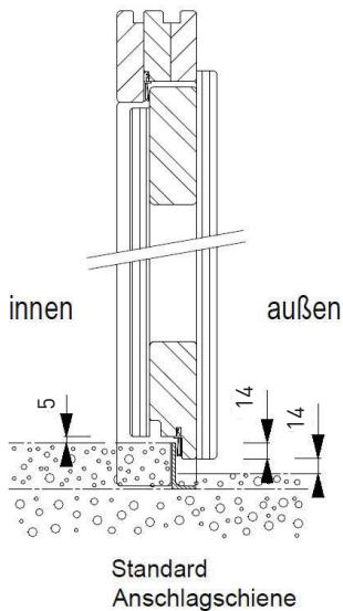
T20 beidseitig verschalt nach außen aufgehend
