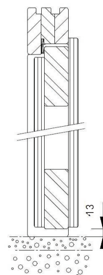
T20 ohne Bodenschiene
