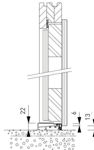
T20 Profilschwelle nach außen aufgehend
